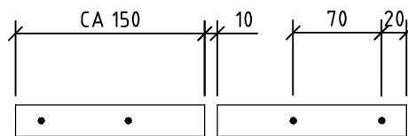
FIG 1 - PLAN BANDSTÅL 2+2 HÅLØ5
