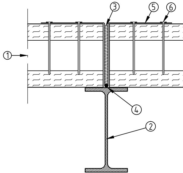
FÖRANKRING I STÅLBALK
